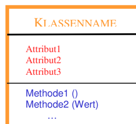
Klassendiagramm
