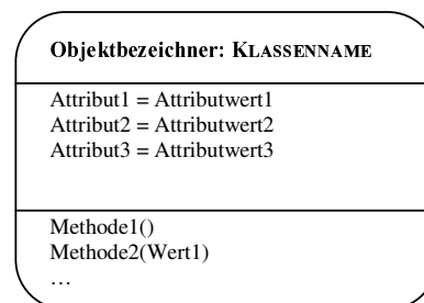
Objektdiagramm
